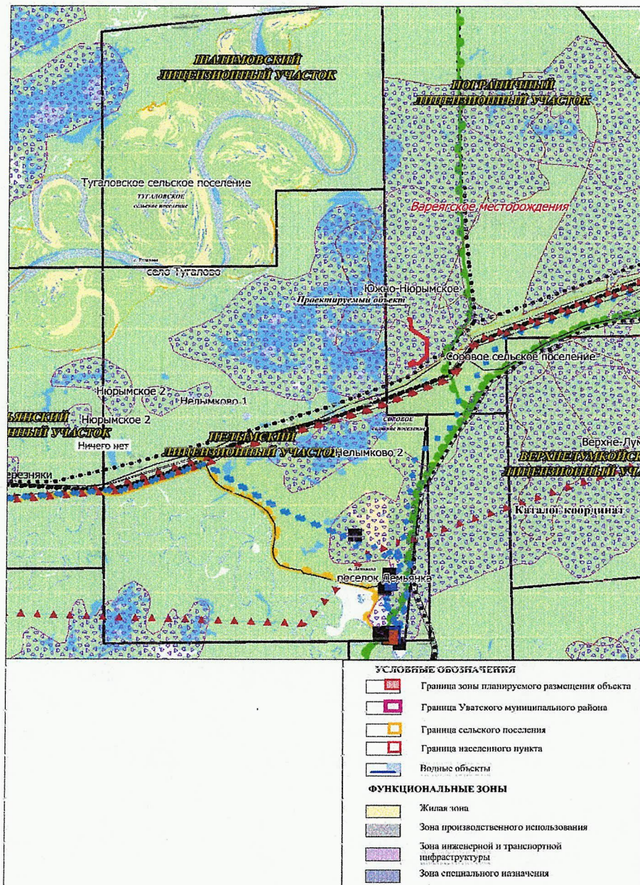
Обзорная схема по проекту: «Обустройство кустовой площадки № 5. Варягского месторождения нефти Пограничного лицензионного участка. Корректировка».
